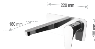
L 15 Miscelatore monocomando a incasso per lavabo, con piastra rettangolare in ottone cromato. Single-lever built-it basin mixer, with rectangular wall flange in chrome plated brass.
